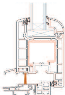
Coupe verticale 20 mm Partie ouvrante
